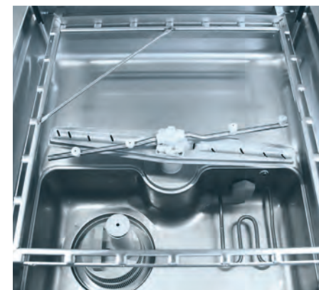
UPster H 500 Syvävedetty pesutankki sijaitsee koneen edessä. Tankki on suunniteltu siten, että se on helppo huoltaa ja on helppopääsyinen. Yksi erityinen etu on se, ettei koneen sisäosan takaseinässä ole käyttöä ja huoltoa häiritseviä letkuja ja putkia. Erittäin käyttäjäystävällinen EcoFilter –suodatinjärjestelmä.
