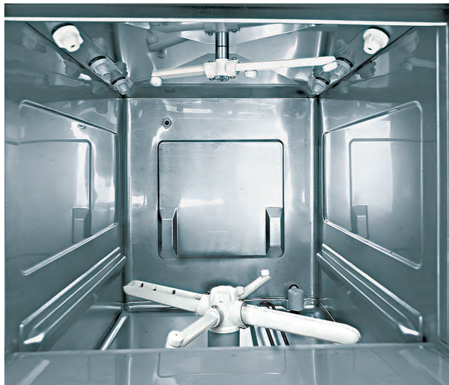
UPster U 400 Kauniisti muotoiltu pesukammio ammattimaiseen käyttöön: lujatekoinen teknologia ja korkealuokkaiset materiaalit takaavat erinomaisen pesutuloksen vain 11 litran tankkitäytöksellä.
