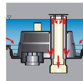
Alkuperäinen Meiko EcoFilter –järjestelmä suodattaa tankkivettä tehokkaasti maksimoiden hygienian ja tankkiveden puhtauden.
